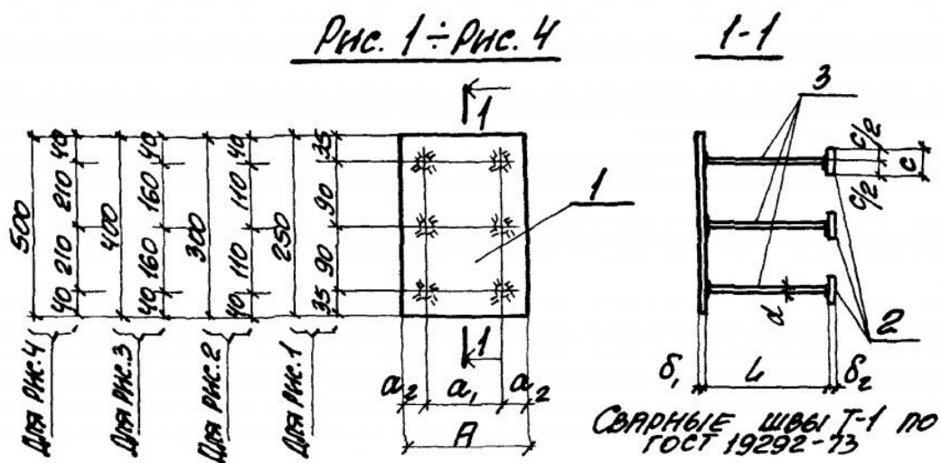
Чертеж 1. Закладные детали МН133-МН145
