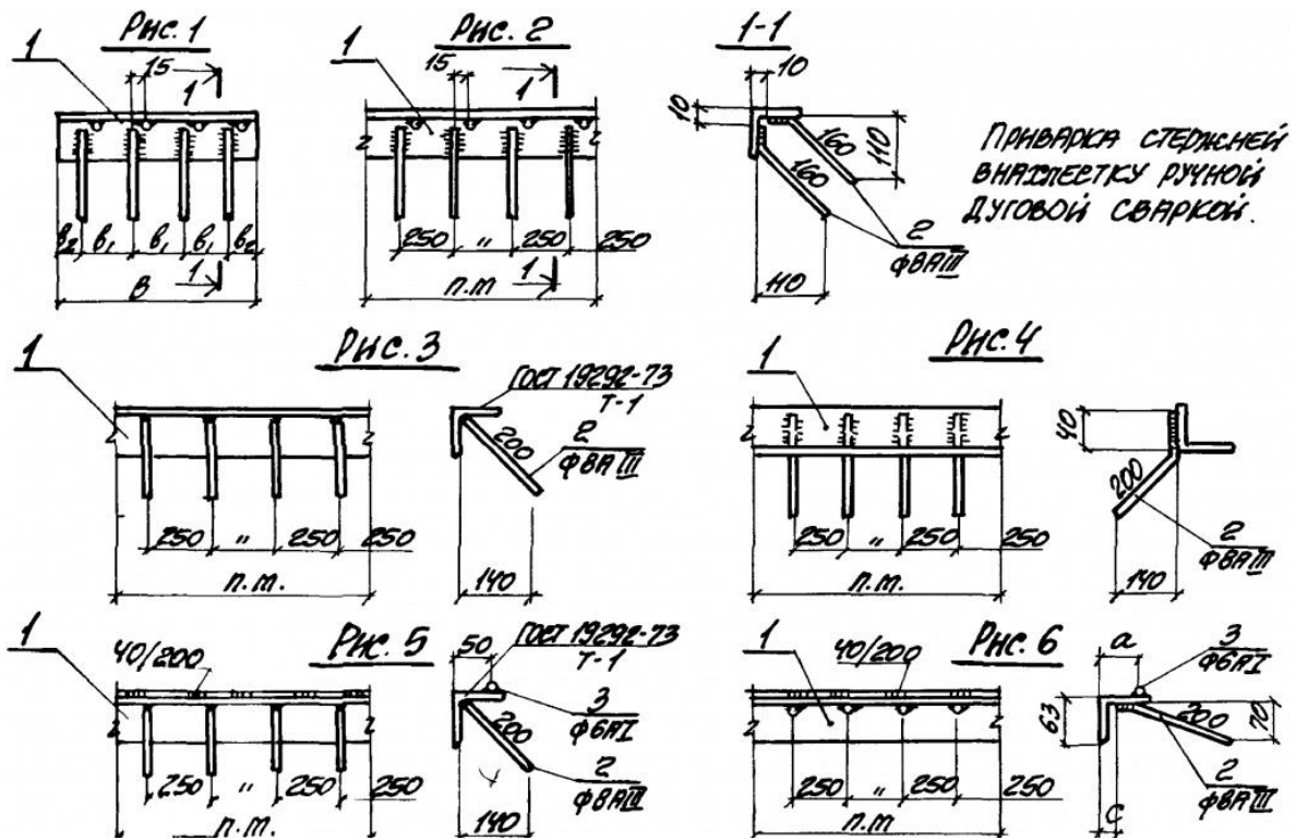
Чертеж 1. Закладные детали МН549-МН577
