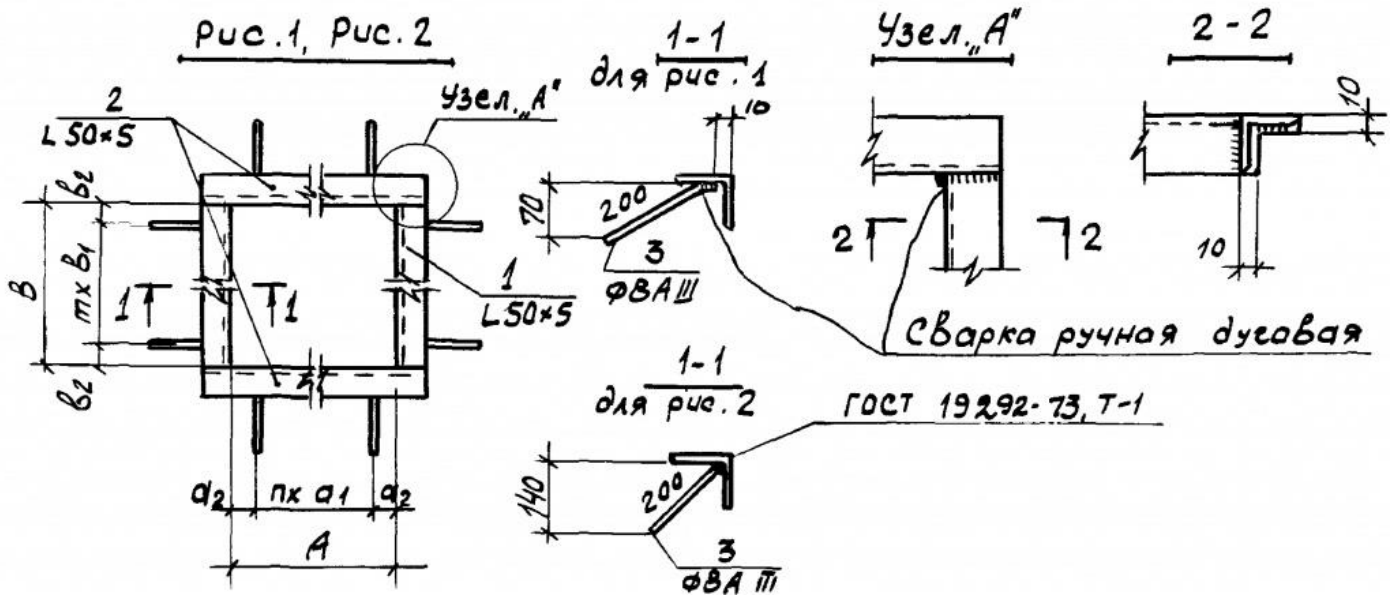
Чертеж 1. Закладные детали МН726-МН775
