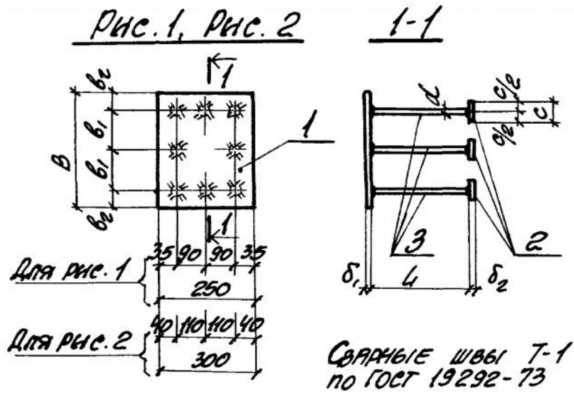
Чертеж 1. Закладные детали МН146-МН151
